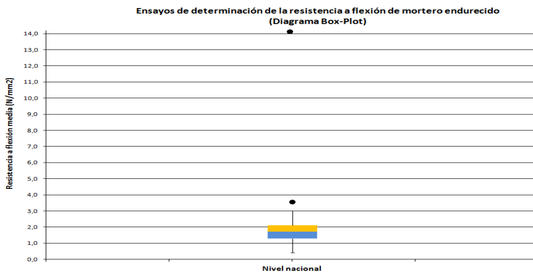
Gráfico. Diagrama de cajas del ensayo de determinación de la resistencia a flexión
