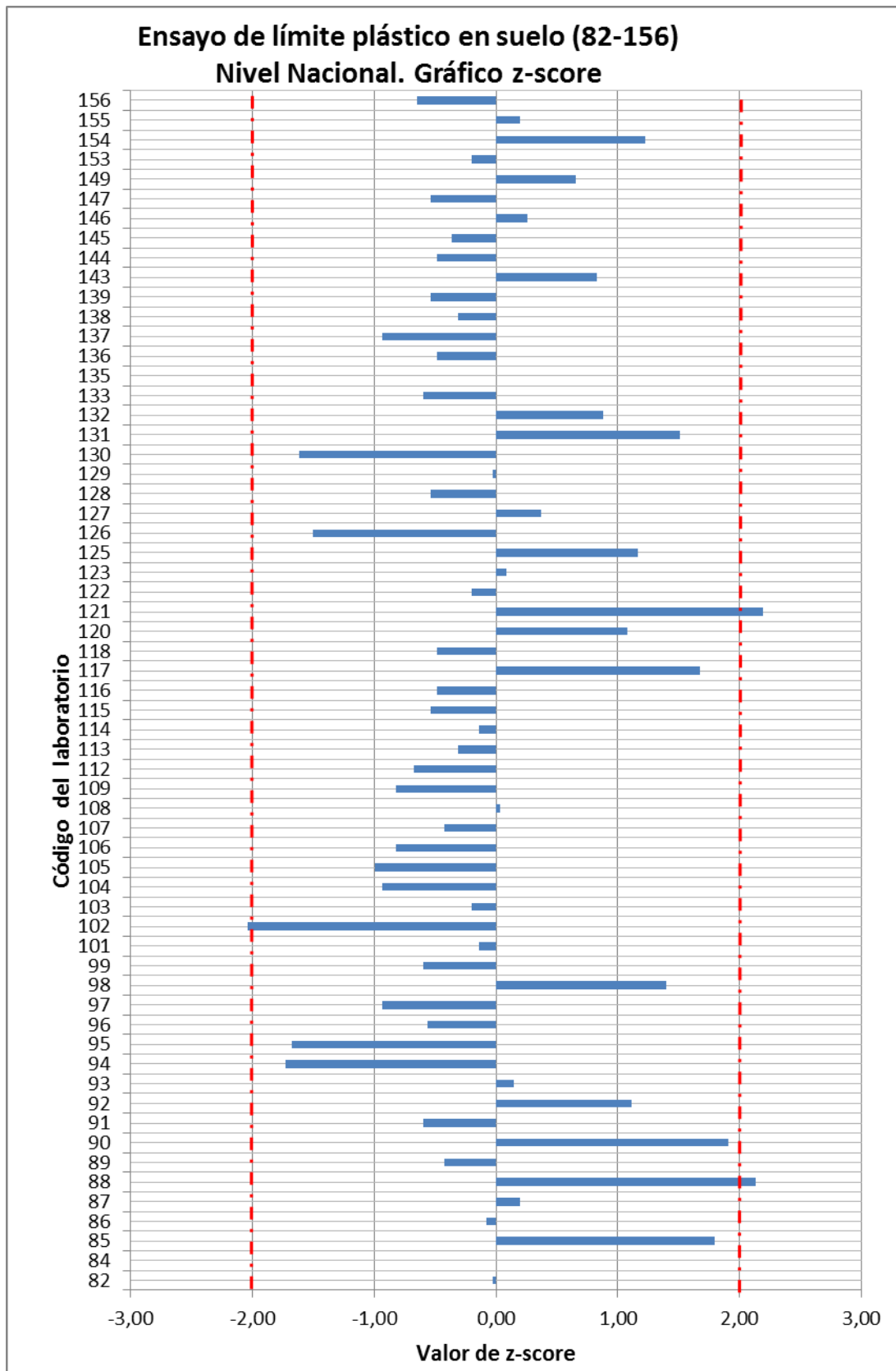
Gráfico 3b. Valores de z-score del ensayo de límite plástico a partir de resultados por laboratorio a nivel nacional.
